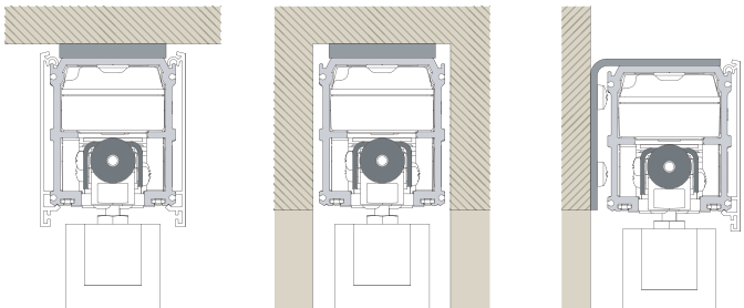
DECKENBEFESTIGUNG
